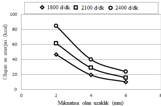
Şekil 5. Mıknatısa olan uzaklık ile sistemde üretilen ısı enerjisinin değişimi
