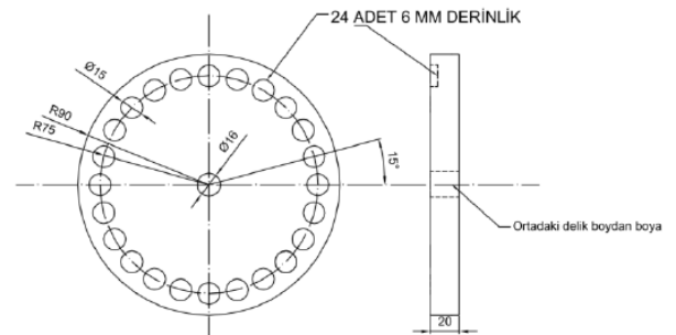
Şekil 3. Mıknatıs dizili rotorun çizimi
