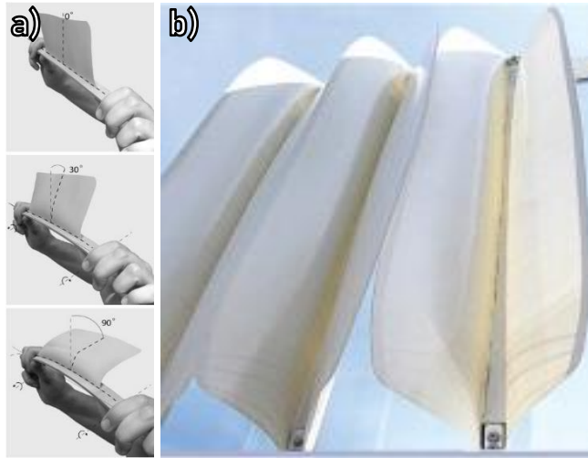
Şekil 9. Flectofin®'nin; (a) cennet kuşunun çiçeğinden esinlenilen hareket prensibi, (b) örnek uygulaması (Kaynak: (a) Lienhard vd., 2011, (b) Schleicher vd., 2015)
