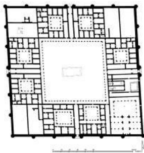
Şekil 1 (solda) Kasrû’l Hayri-ş Şarkî (Anonim, tb: 8) Şekil 2 (ortada ve sağda) Kasrû’l Tuba (Sanatın yolculuğu, 2019)
