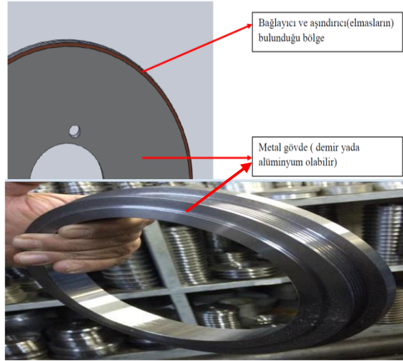
Şekil 2. Rodaj disk yapısı
