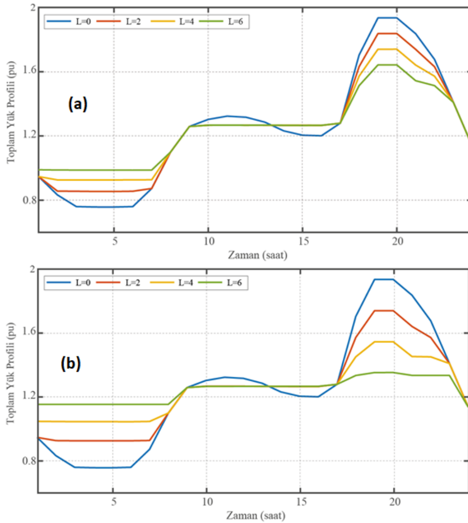
Şekil 5. 9 Baralı bir dağıtım sisteminde |L| = 0, 2, 4, 6 enerji depolama sistemi sayıları için üretim profili. (a) Enerji depolama sistemi kapasitesi sistemin maksimum talep değerinin %10'u olduğunda toplam yük profilindeki değişim. (b) Enerji depolama sistemi kapasitesi sistemin maksimum talep değerinin %20'si olduğunda toplam yük profilindeki değişim.
