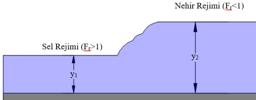
Şekil 4. Hidrolik sıçramanın genel şeması.
