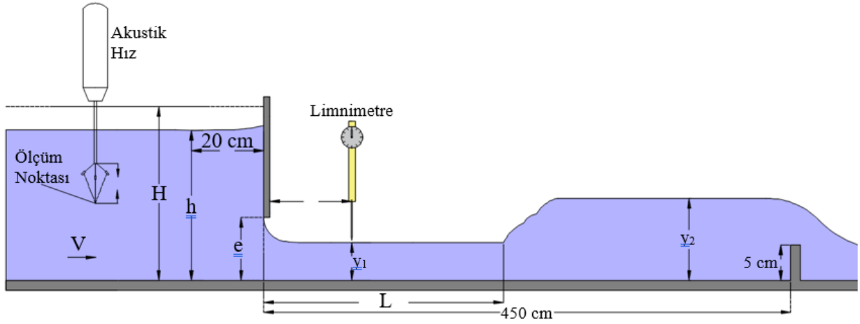
Şekil 7. Fiziksel deney düzeneğinin genel görünümü ve ölçüm yapılan noktalar.
