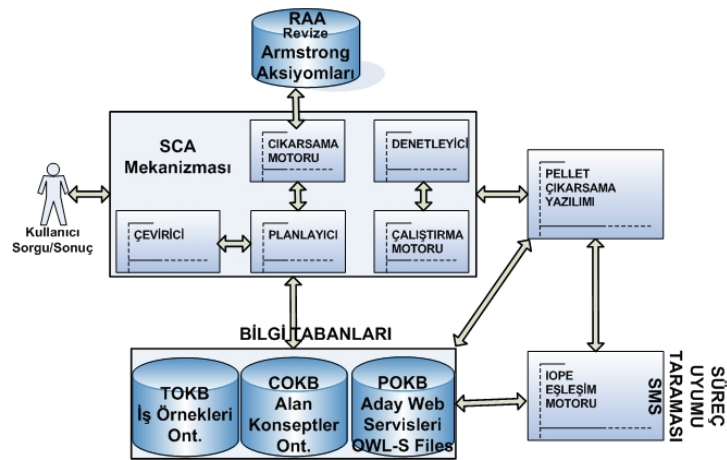
ŞEKİL 2. SCA sisteminin genel mimarisi.
