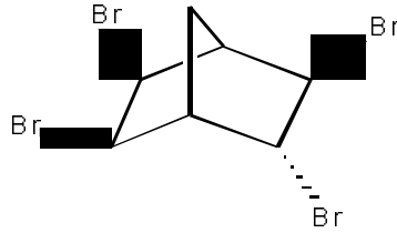
Şekil 1. C 7 H 8 Br 4 molekülün kimyasal formülü.
