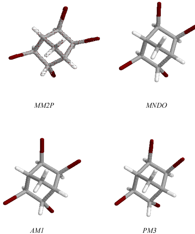
Şekil 2. C 7 H 8 Br 4 'in MM2P ve yarı-deneyssel kuantum mekanik MNDO, AM1 ile PM3 yaklaşım yöntemleri ve X-ışınları analizi sonucu elde edilen deneyssel verilerle çizilen uzaysal görünüşleri.
