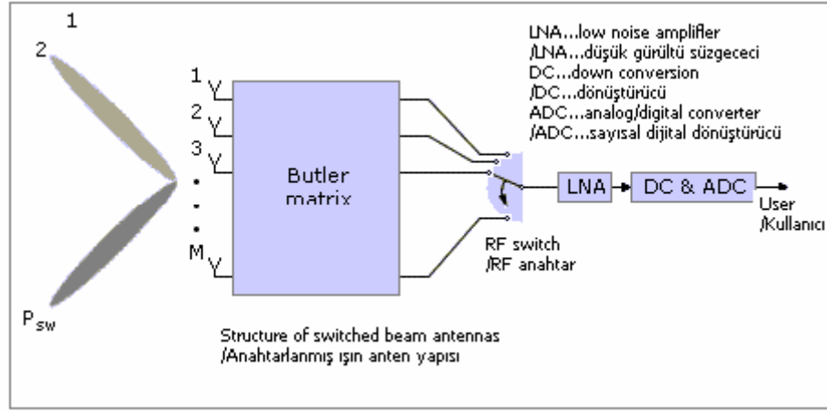
Figure 8. Hardware structure of a receiver with RF-beamforming - "switched beam antenna" Şekil 8. RF ışın şekillendirici alıcının donanım yapısı "Anahtarlama Işın Anten"
