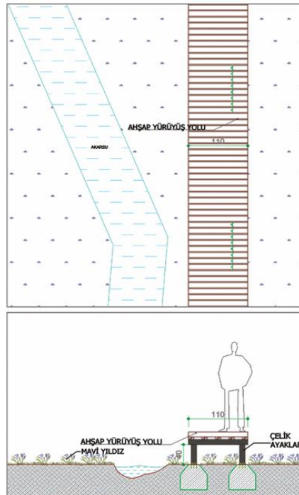
Şekil 8. Önerilen Ahşap Yürüyüş Platformu Plan-Kesit
