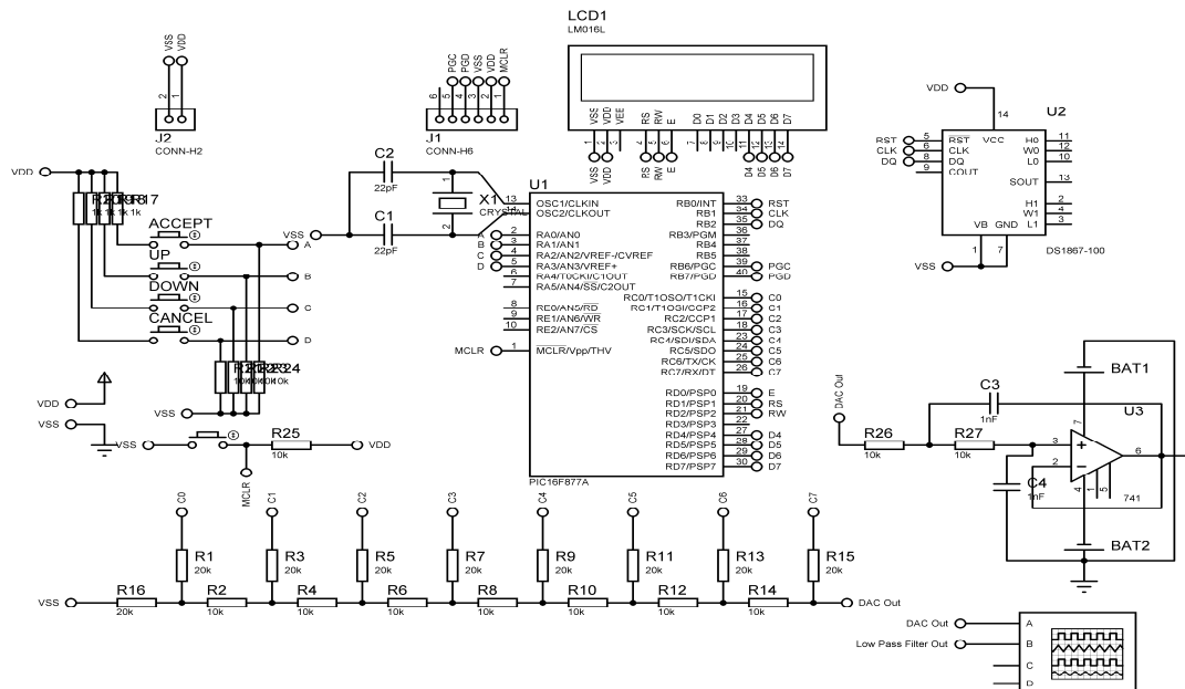
Fig. 6. Circuit Schema
