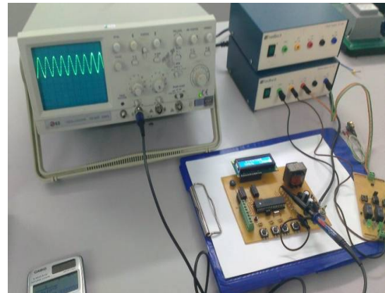
Fig. 8. Sinus wave output
