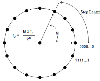
Fig. 3. Phase Circle
