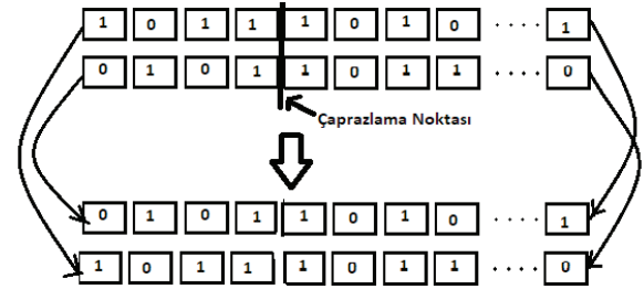
Şekil 3. Genetik algortmada çaprazlama örneği
