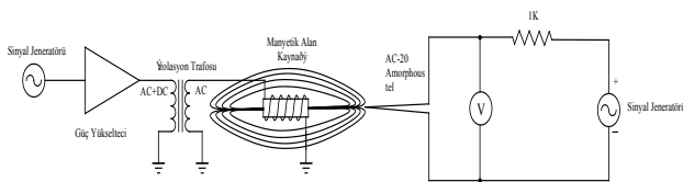
Şekil 8. GMI sensör ile uzaktan algılama
