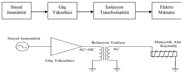
Şekil 2. Manyetik alan kaynağının blok diyagramı ve açık şeması
