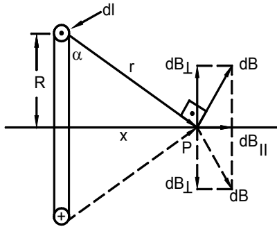
Şekil 6. Bir halkanın kendisinden x kadar uzakdaki manyetik akı yoğunluğu
