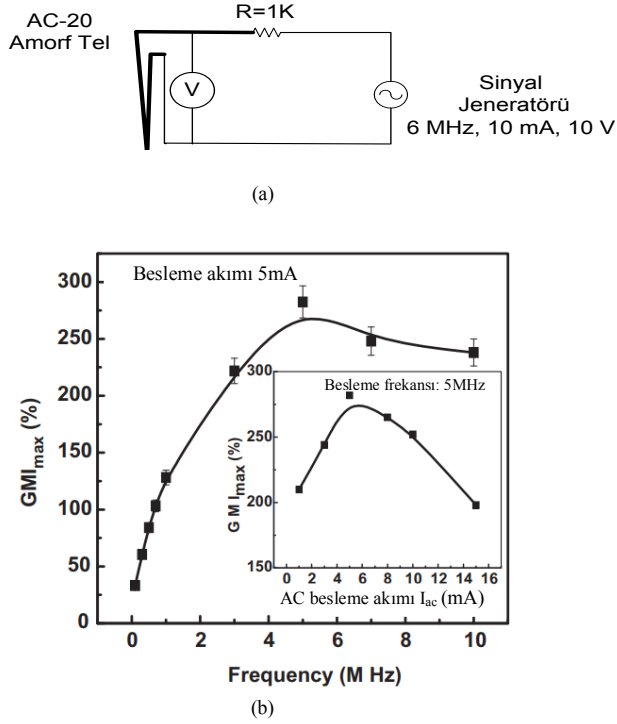
Şekil 1. Amorf telin manyetik sensör olarak kullanımı[8,9]
