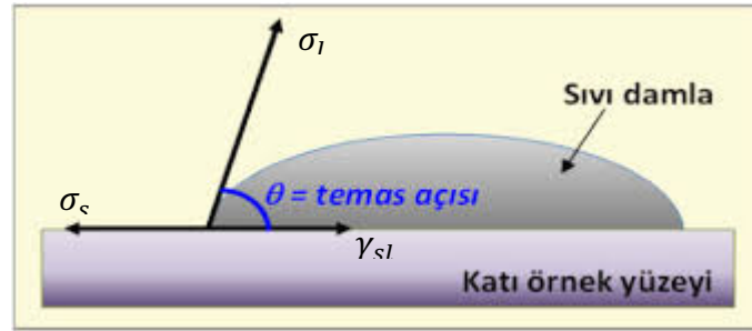
Şekil 2.Katı sıvı ara yüzeyinde temas açısının oluşumu
