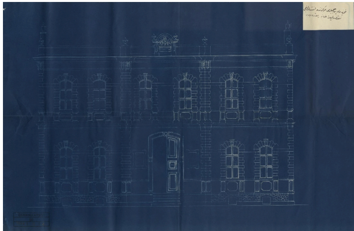
Görsel 2: Konya Vilayeti Telgraf ve Postahane binası ana cephe çizimi Kaynak: BOA. ŞD. 1130/11
