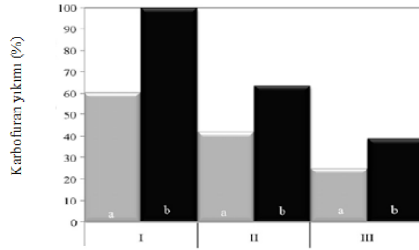
Şekil 3.2. Ultrases/Fenton prosesinin karbofuran yıkımına olan etkisinin başlangıç konsantrasyonuna göre belirlenmesi [ \text{Fe}^{2+} : 10 mg/L, \text{H}_2\text{O}_2 : 100 g/L; (a) Fenton prosesi; (b) Ultrases+ Fenton prosesi; Karbofuran konsantrasyonu I: 20 mg/L; II: 100 mg/L; III: 200 mg/L] (Ying-Shih ve ark., 2010)
