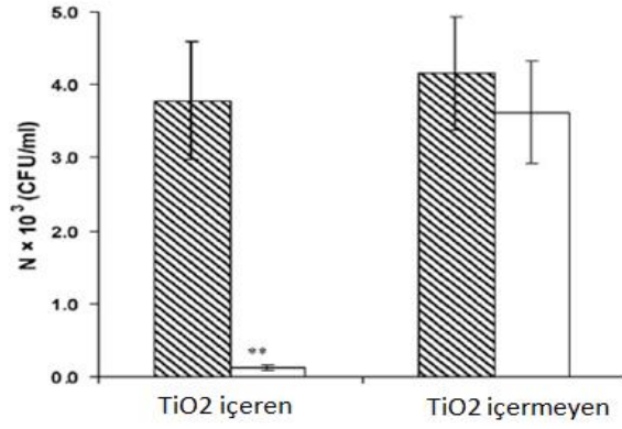
Şekil 2.3. TiO 2 in Legionella hücrelerine olan etkisi. (Gölge sütunlar uygulama öncesi; açık renkli sütunlar ise 30dk'lık ultrases uygulaması ve 1.0g/ml derişimlerde TiO 2 uygulamalarını göstermektedir) (Shimizu ve ark., 2010).
