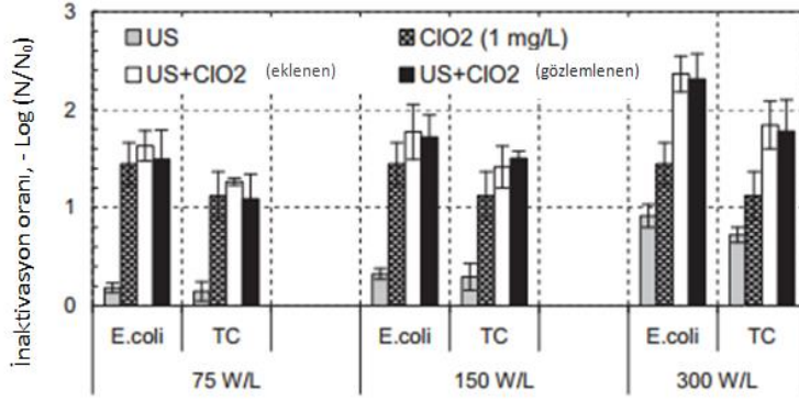
Şekil 2.1. E.coli ve Total Koliform (TC) üzerine Ultrases, \text{ClO}_2 'nin ayrı ayrı ve birlikte etkisi (Ayyıldız ve ark., 2011)
