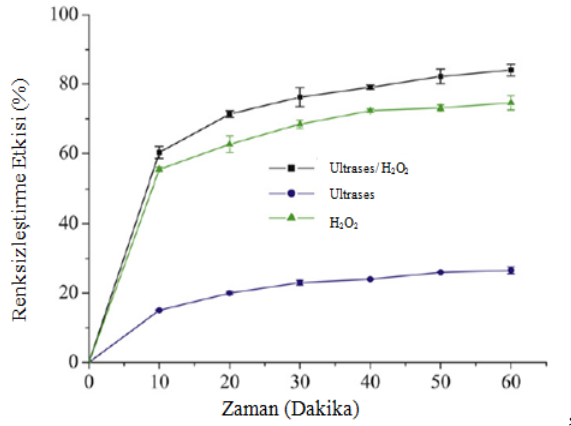
Şekil 2.4. Farklı renksizleştirme yöntemlerinin karşılaştırılması; Ultrases, H_2O_2 ve Ultrases, H_2O_2 . ( Cyclocarya paliurus (Batal.) Iljinskaja polisakkaritlerinin konsantrasyonu, 0.5 mg/ml; H_2O_2 , 0.623 mM; Sıcaklık 40°C; Uygulama Süresi 60 dakika) (Xie ve ark., 2011)
