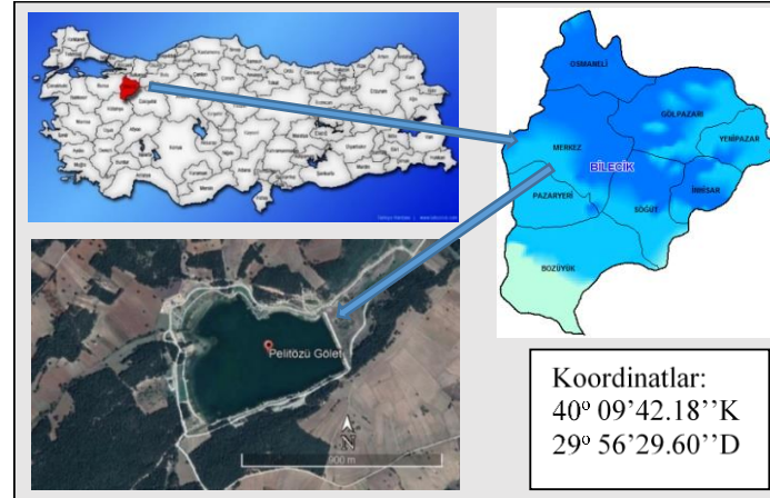
Şekil 1. Çalışma alanı
