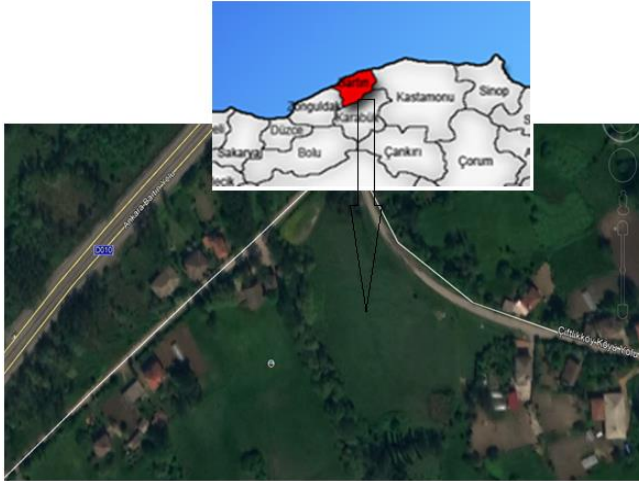
Şekil 1. Bartın'ın Türkiye haritasındaki yeri ve araştırma alanına ait uydur görüntüleri
