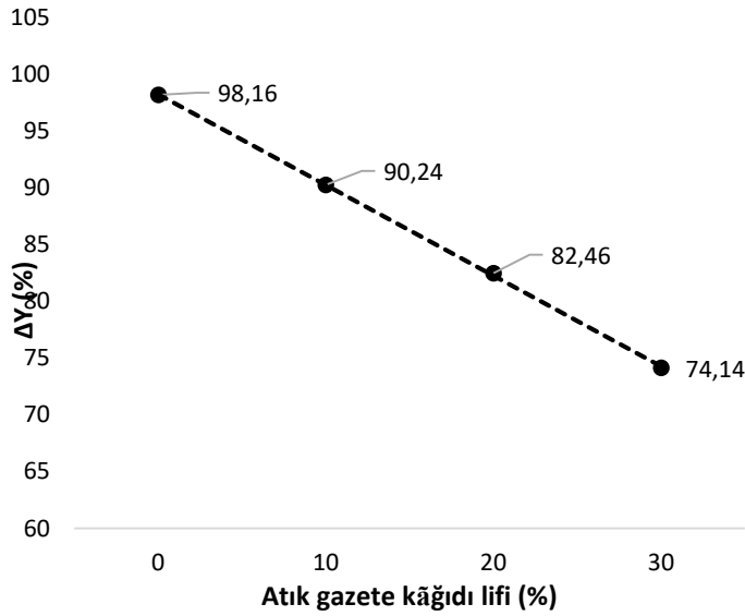
Şekil 6. Lif miktarının ΔY değeri üzerine etkisi
