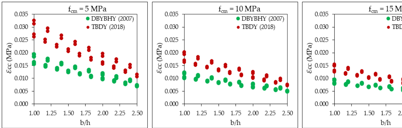
Şekil 9. 3 kat lifli polimerle sargılanan kesitlerin birim şekil değiştirme değerleri.
