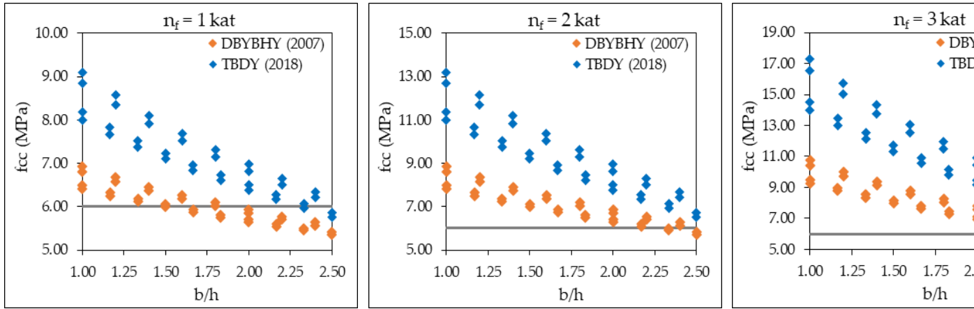
Şekil 4. 5 MPa beton dayanımına sahip kesitlerin lifli polimerle sargılama sonucu beton basınç dayanımları.
