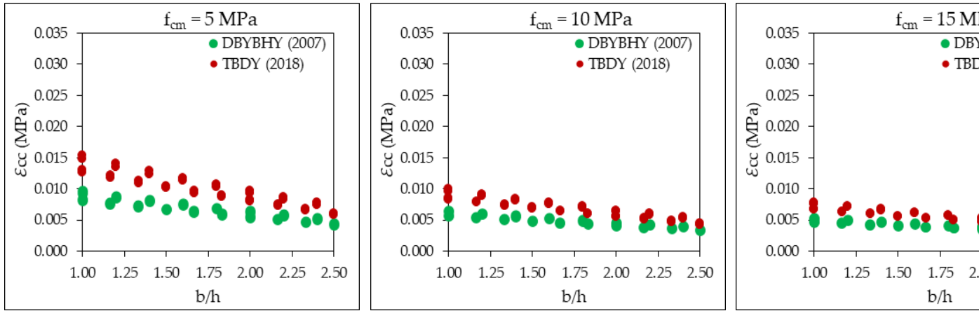
Şekil 7. 1 kat lifli polimerle sargılanan kesitlerin birim şekil değiştirme değerleri.
