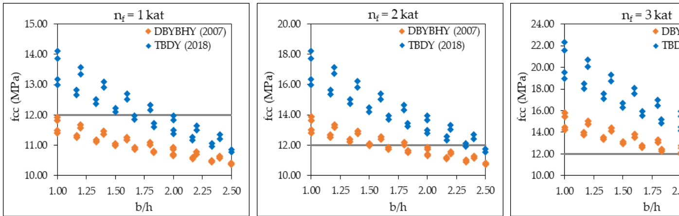
Şekil 5. 10 MPa beton dayanımına sahip kesitlerin lifli polimerle sargılama sonucu beton basınç dayanımları.
