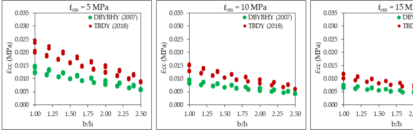
Şekil 8. 2 kat lifli polimerle sargılanan kesitlerin birim şekil değiştirme değerleri.
