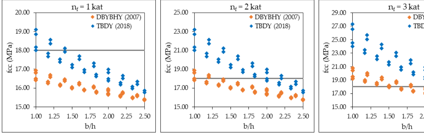
Şekil 6. 15 MPa beton dayanımına sahip kesitlerin lifli polimerle sargılama sonucu beton basınç dayanımları.
