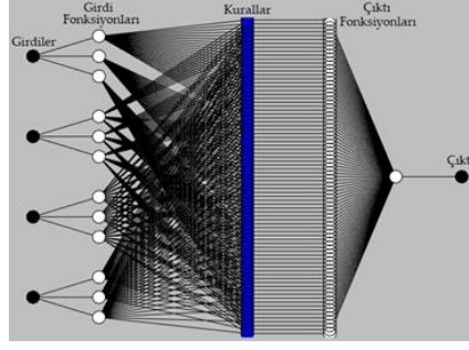
Şekil 3. Anfis modellerinin yapısı.
