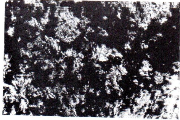
Resim 8: 60 dakika etching işlemi yapılan Cr-Co alaşımı. Büyütme x 600.
