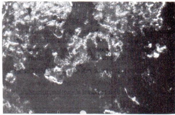
Resim 4: 60 dakika etching işlemi yapılan Cr-Ni alaşımı. Büyütme x 600.
