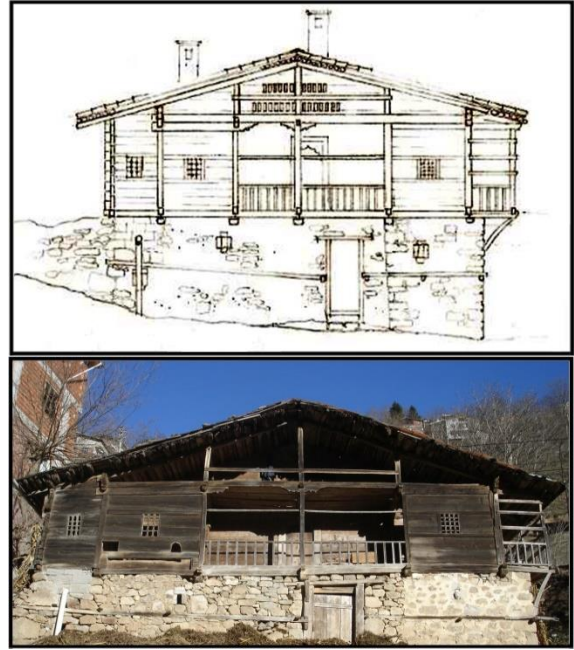
Şekil 4. Ahşap yığma sistemi ile yapılan konutların cepheleri, (Taşkiran-Trabzon Koruma Amaçlı Uygulama İmar Planı Raporu Kutluay Planlama, Z. Özcan Bölümü, 2012-2013).
