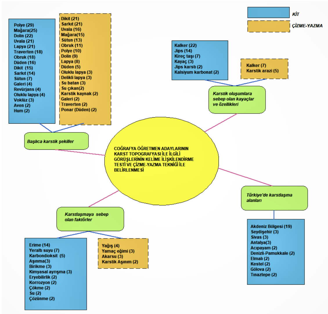
Şekil 2: Coğrafya Öğretmen Adaylarının Karst Topografyası Anatar Kavramıyla İlgili Bağımsız Kelime İlişkilendirme Testi ve Çizme-Yazma Tekniği ile Belirlenen Bilişsel Yapılarının Modeli
