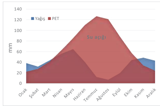
Şekil 4: Thornthwaite Su Bilançosu (Tokat İstasyonu)
