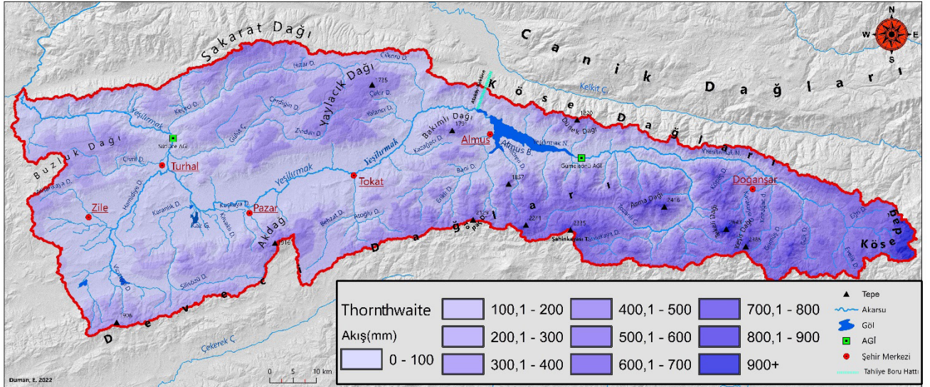
Şekil 5: Çalışma Sahasının Thornthwaite Yöntemine Göre Oluşturulan Akış Haritası.
