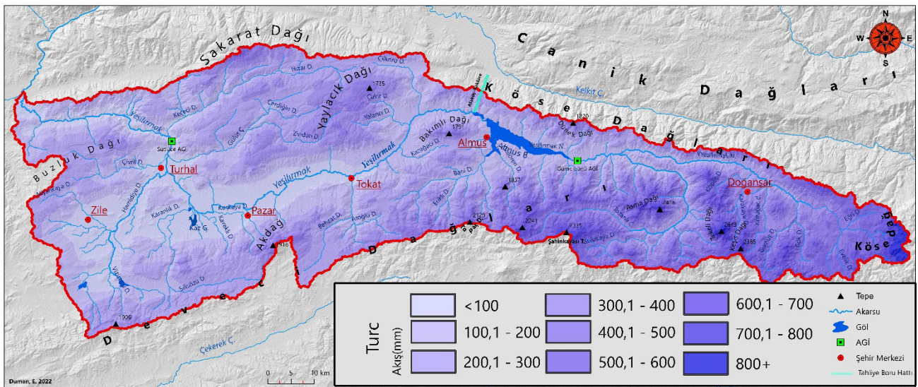
Şekil 6: Çalışma Alanının Turc Yöntemine Göre Oluşturulan Akış Dağılım Haritası.
