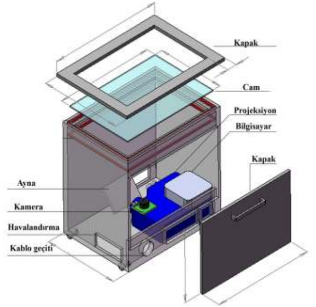
Şekil 5. Sistem düzeneği
