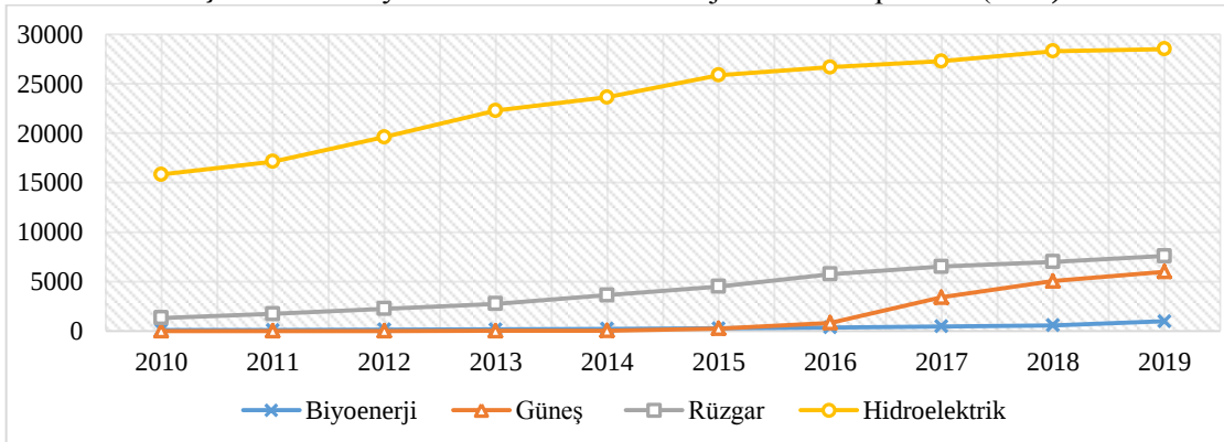
Şekil 7. Türkiye'nin Yenilenebilir Enerji Kurulu Kapasitesi (MW)
