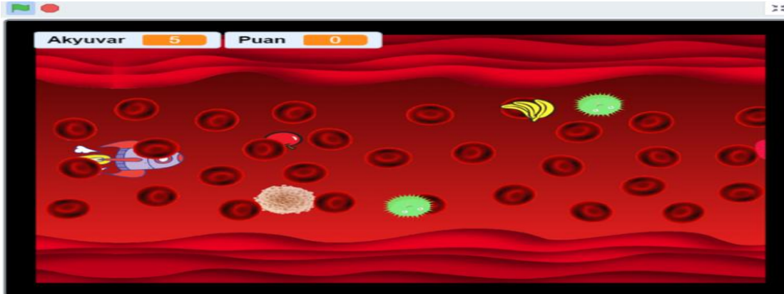
Şekil 3. Kan damarı içinde hareket simülasyonu
