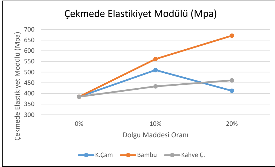
Şekil 6. Üretilen Örneklerin Çekmede Elastikiyet Modülü Etkileşim Grafiği
