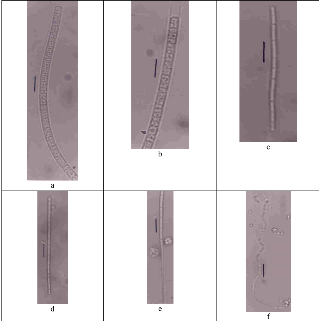
Şekil 4.a- Oscillatoria tenuis C.A. Agardh b- Phormidium ambiguum Gomont c- Phormidium mucicola Noumann d- Phormidium tenue (Menegh.) Gomont e- Lyngbya lagerheimi Gomont f- Lyngbya versicolor Wartmann ex Gomont (Ölçüler 10µm)
