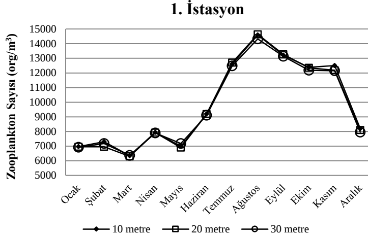
Şekil 8. 1. istasyon (deniz bölgesi)'nda 10, 20 ve 30 metre derinliklerdeki zooplankton yoğunlukları( \text{org/m}^3 )
