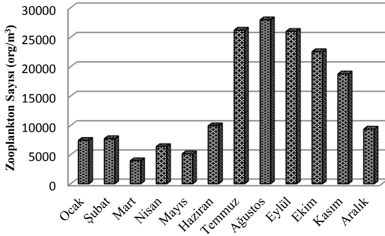
Şekil 9. Toplam zooplankton yoğunluğunun aylara göre değişimi ( \text{org/m}^3 )
