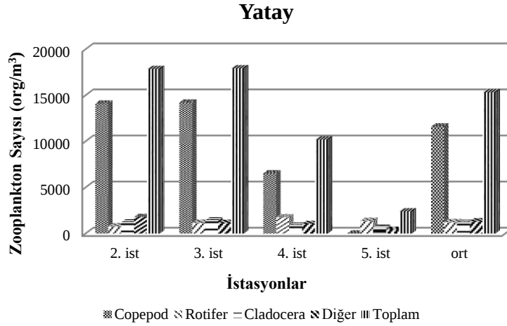
Şekil 6. Manavgat Nehri nehirağzı bölgesi 2.,3.,4. ve 5. istasyonlarda (deniz bölgesi hariç) yatay çekimler sonucu elde edilen zooplankton gruplarının ortalama yoğunluğu ( \text{org/m}^3 )
