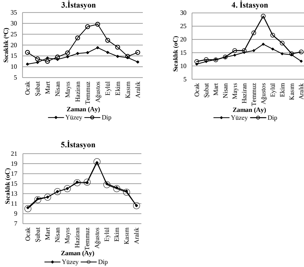
Şekil 2. Manavgat Nehri nehiragzı bölgesi yüzey ve dip suyu sıcaklık değerleri (°C)
