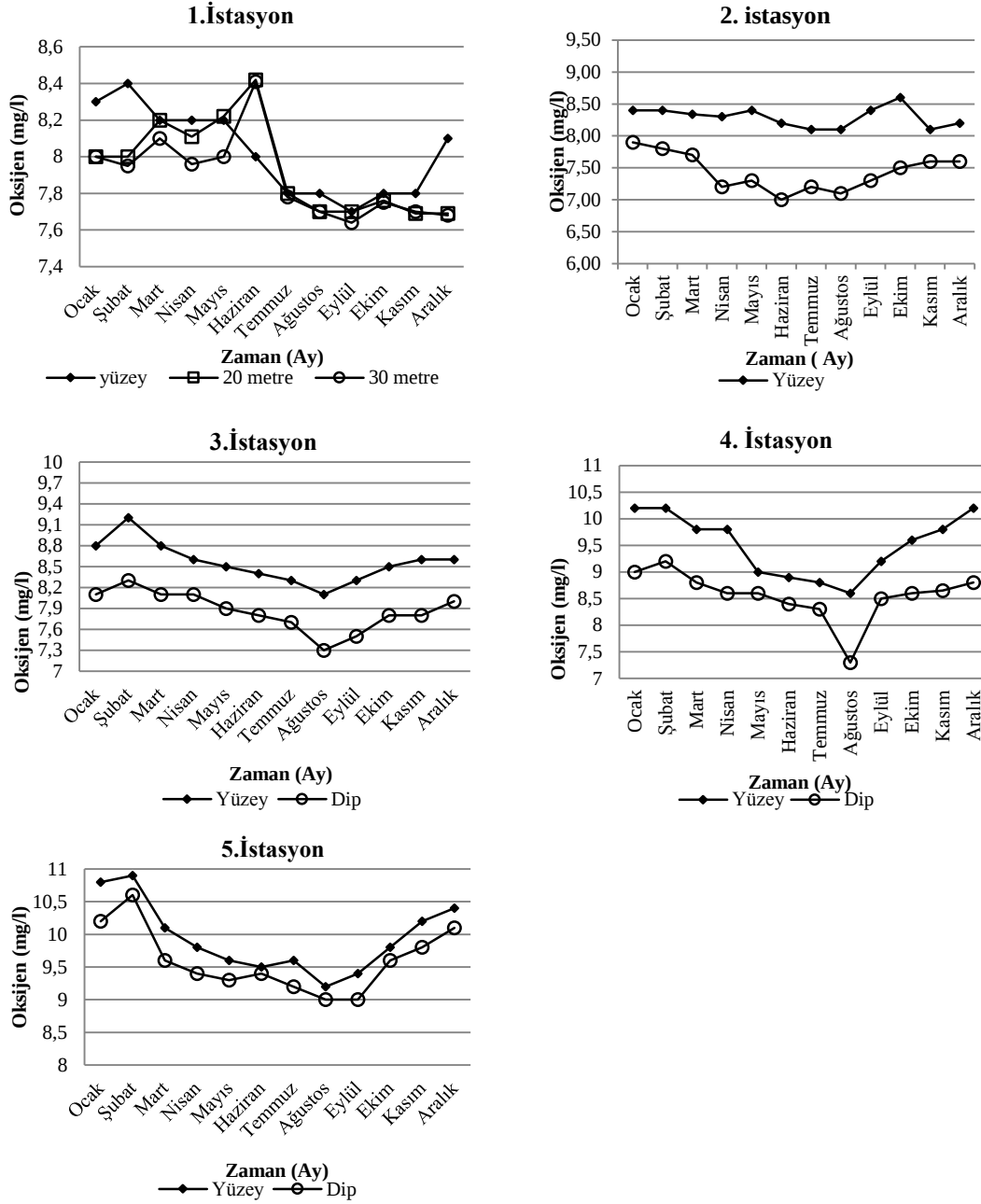
Şekil 4. Manavgat Nehri nehirağzı bölgesi yüzey ve dip suyu çözünmüş oksijen değerleri (mg/l)
