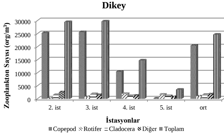
Şekil 7. Manavgat Nehri nehirağzı bölgesi 2.,3.,4. ve 5.istasyonlarda (deniz bölgesi hariç) yatay çekimler sonucu elde edilen zooplankton gruplarının ortalama yoğunluğu ( \text{org/m}^3 )
