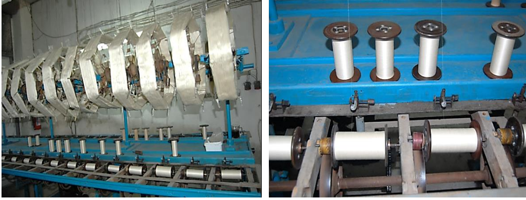
Şekil 0-1 İpek ipliğinin cam kılavuzlar yardımıyla çileden makaralara aktarılması (N.G.Değerli, Ödemiş, 2012)
