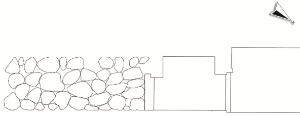
Çizim 1. Mezarın AA Kesiti
