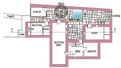
Plan 23. Saim Sakaoglu Evi Zemin Kat Planı (Arat, 2018).
