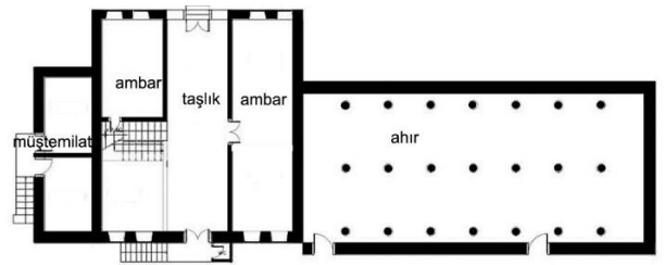
Plan 5. Demiralay Konağı Zemin Kat Planı (Akan ve Örmecioğlu, 2016).
