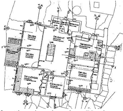
Plan 2. Müftüoğlu evi üst kat planı (Hacıkura, 2000).
