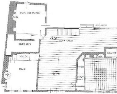
Plan 11. Hacı Efendi Evi Esas Kat Planı (Minez, 2006).
