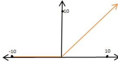
Şekil 4. Relu fonksiyonun grafiği
