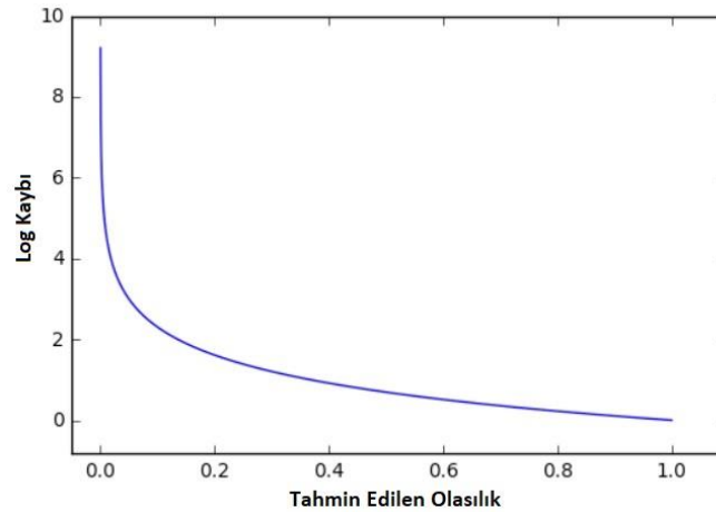
Şekil 5. Gerçek değer 1 iken log kaybı grafiği (Fortuner, 2019).
