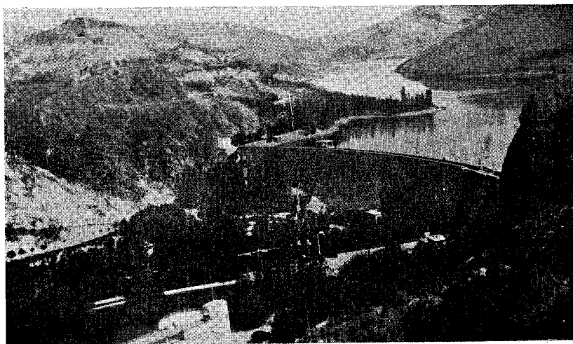
Fig. 1, Vue sur la digue du barrage de Tehouabouk
