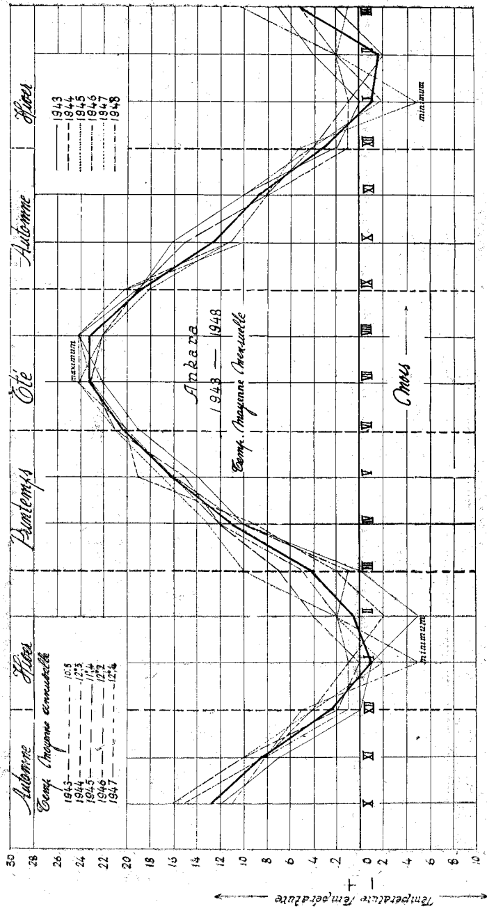
Courbes indiquant la température moyen, mensuel : (1943-48)
