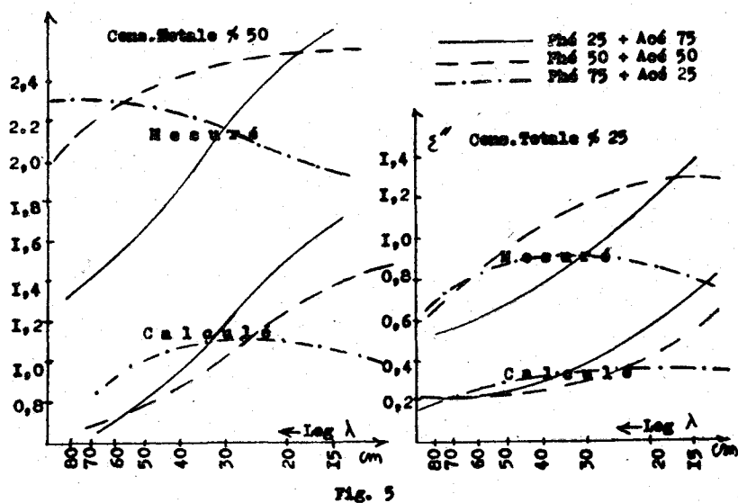
Fig. 5 Comparation des valeurs mesurées et calculées \epsilon' et \epsilon'' des mélanges des solutions de Phénole et d'Acétophénone
