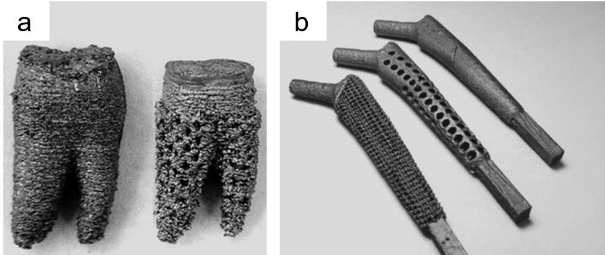
Şekil 18: Farklı gözeneklilik oranlarında NiTi implantlar a) diş implantları ve b) kalça eklem implantları [55-57]
