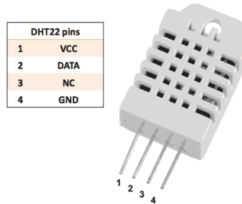
Şekil 2. DHT22 Sensörüne ait pin yapısı ve teknik özellikleri
