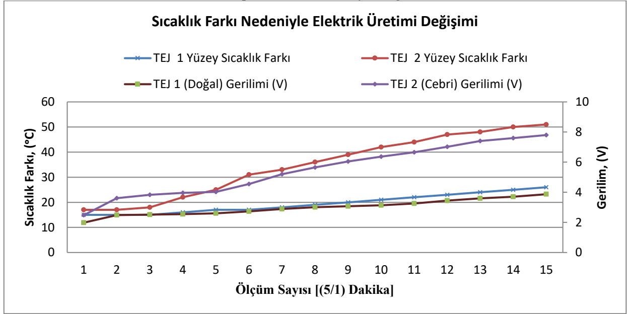
Şekil 14: Deney 2 TEJ Sıcaklık Farkı Elektrik üretimi
