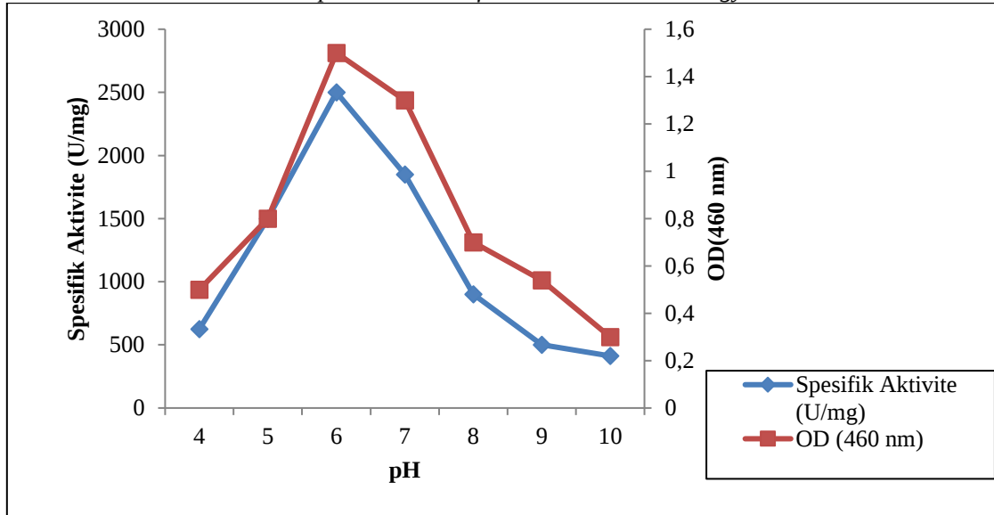
Şekil 4. pH'nın bakteri gelişimi ve enzim üretimine etkisi
