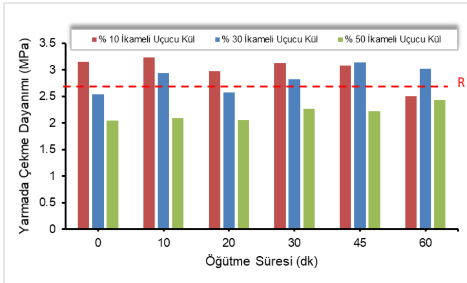
Şekil 6. Yarmada Çekme Dayanımı Sonuçları.
