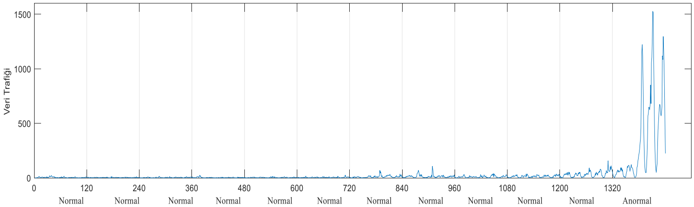
Şekil.3.Verilerin pencereleme bölünmesi
