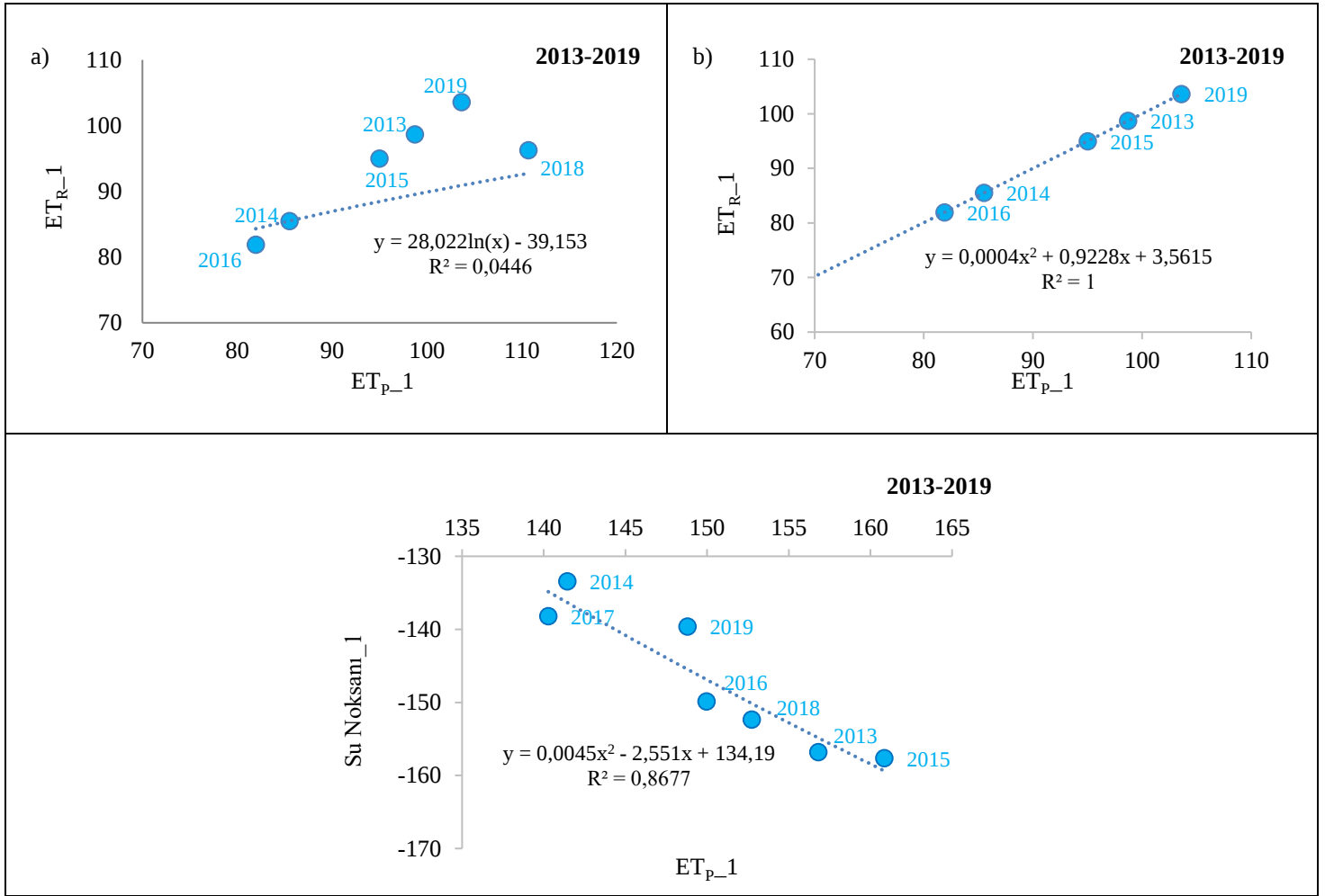
Şekil 13. Yağışlı dönem 2013-2019 yılları arasındaki ET p1 -ET R1 (a), 2013-2019 yılları arasındaki (2017-2018 hariç) ET p1 -ET R1 (b) ve 2013-2019 yılları arasındaki Su Noksani 1 -ET p1 (c) ilişkisi
