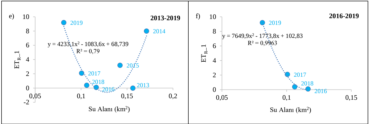
Şekil 10. Kurak dönemde 2013-2019 yılları arasında NDWI ile belirlenen su alanı ile SPI1 (a) 2016-2019 yılları arasında alan ile SPI1 (b), 2013-2019 yılları arasında alan ile ET_{p1} (c), 2013-2019 yılları arasında ET_{R1} ile SPI1 (d), 2013-2019 yılları arasında alan ile ET_{R1} (e) ve 2016-2019 yılları arasındaki alan ile ET_{R1} (f) ilişkisi
