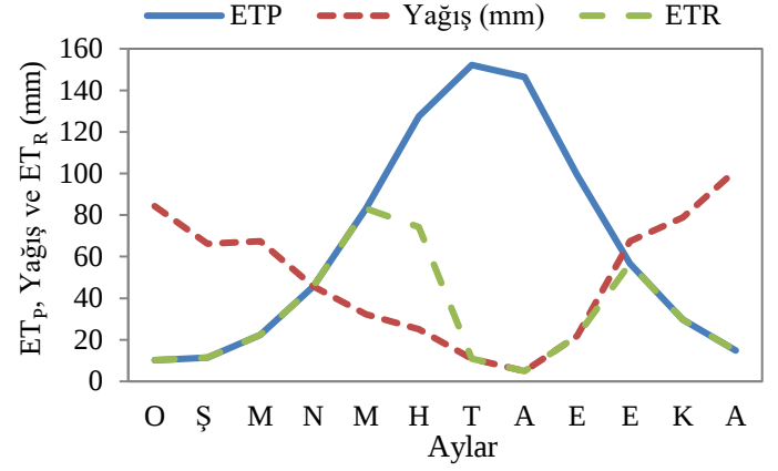
Şekil 8. Lapseki'nin ET_P , Yağış ve ET_R Grafiği
