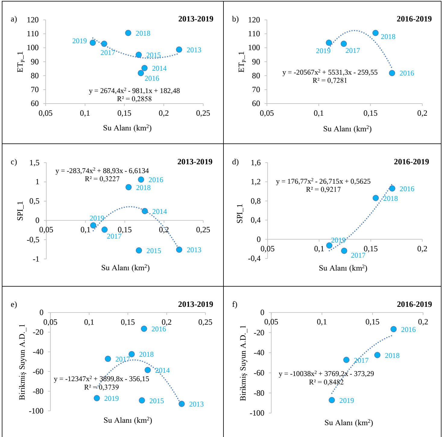
Şekil 12. Yağışlı dönemde 2013-2019 yılları arasında NDWI ile belirlenen su alanı ile ET_p1 (a), 2016-2019 yılları arasındaki su alanı- ET_p1 (b), 2013-2019 yılları arasındaki SPI1 ile su alanı (c), 2016-2019 yılları arasındaki SPI1-su alanı (d), 2013-2019 yılları arasındaki Birikmiş Suyun Aylık Değişimi-1 ile su alanı (e), 2016-2019 yılları arasında Birikmiş Suyun Aylık Değişimi-1 ile su alanı (f) arasındaki ilişki
