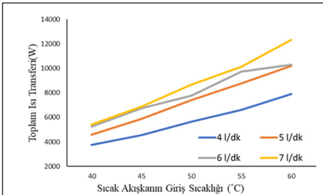
Şekil 8. Farklı Akışkan Debileri İçin Sıcak Akışkan Giriş Sıcaklığına Bağlı Toplam ısı Transferi Miktarı
