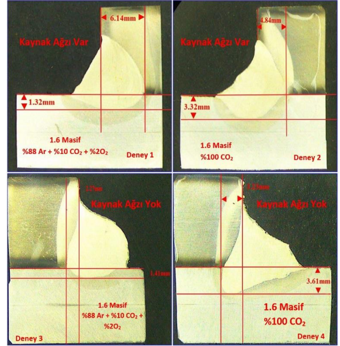
Şekil 7: Makroyapı Görünümleri
