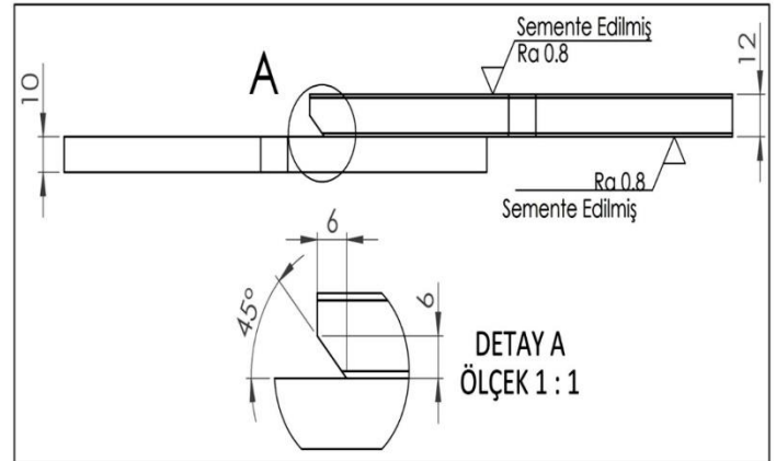
Şekil 4: Deney İşlemine Ait Kaynak Ağzı Açılmış Görünüm
