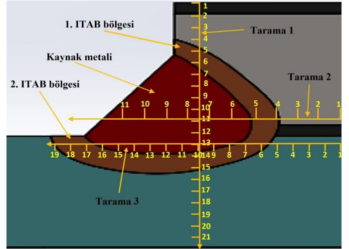
Şekil 8: Sertlik Taramaları
