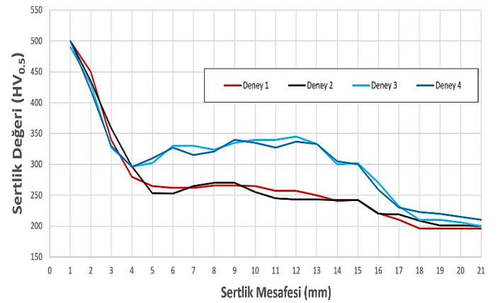
Şekil 9: Tarama 1 Doğrultusuna Ait Sertlik Grafiği
