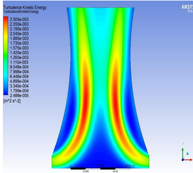
Şekil 8.1. Kule kontrol hacminde kinetik enerji dağılımı (Figure 8.1. Kinetic energy distribution in tower control volume for 1. condit.)
