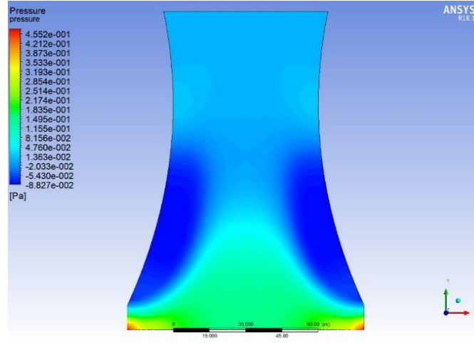
Şekil 7.2. Kule kontrol hacminde basınç dağılımı (Figure 7.2. Pressure distribution in tower control volume for 2. condit.)
