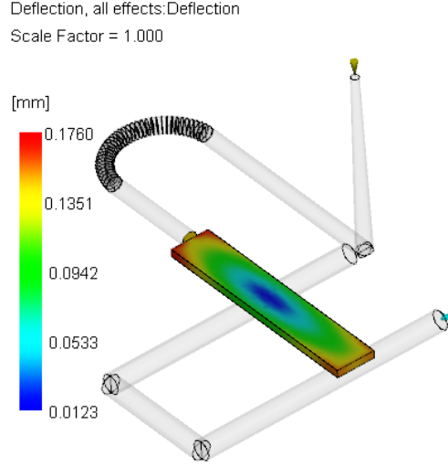
Şekil 3. Hacimsel çekme değerleri
