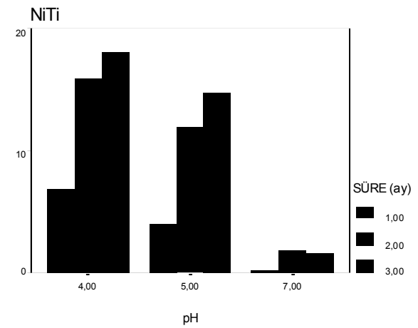
Şekil 7. NiTi ark teline ait pH ve süreye bağlı iyon salınımını gösteren grafik.
