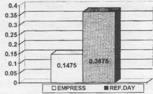
Grafik 2: IPS Empress porselen ve Refraktör day porselen örneklere ait insizal bölgesindeki sızıntı ortalama değerleri
