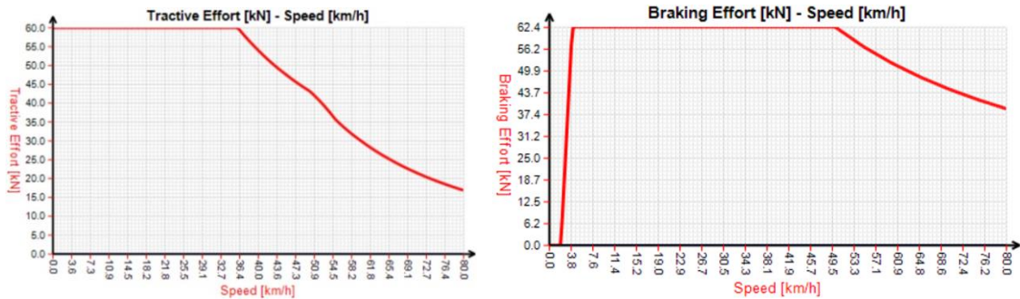
Şekil 4. Trenin cer ve rejeneratif frenleme kuvvet – hız eğrileri. Bir araç için normalize edilmiştir.
